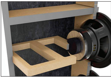
ภาคโครงสร้างอย่างแน่นหนา หนึ่งในระบบขับเคลื่อนสะเทือน DVAS (Driver Vibration Absorption System)
